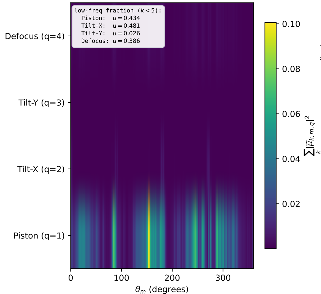
Spectral energy per ray per Zernike mode
